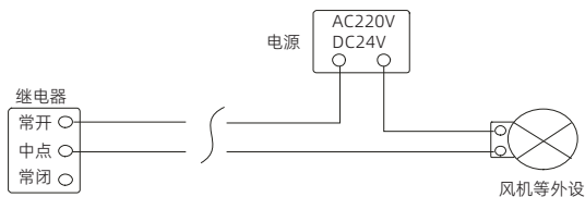
探测器驱动外设参考接线图：
